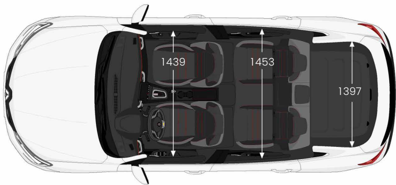
Dimensions (mm).
